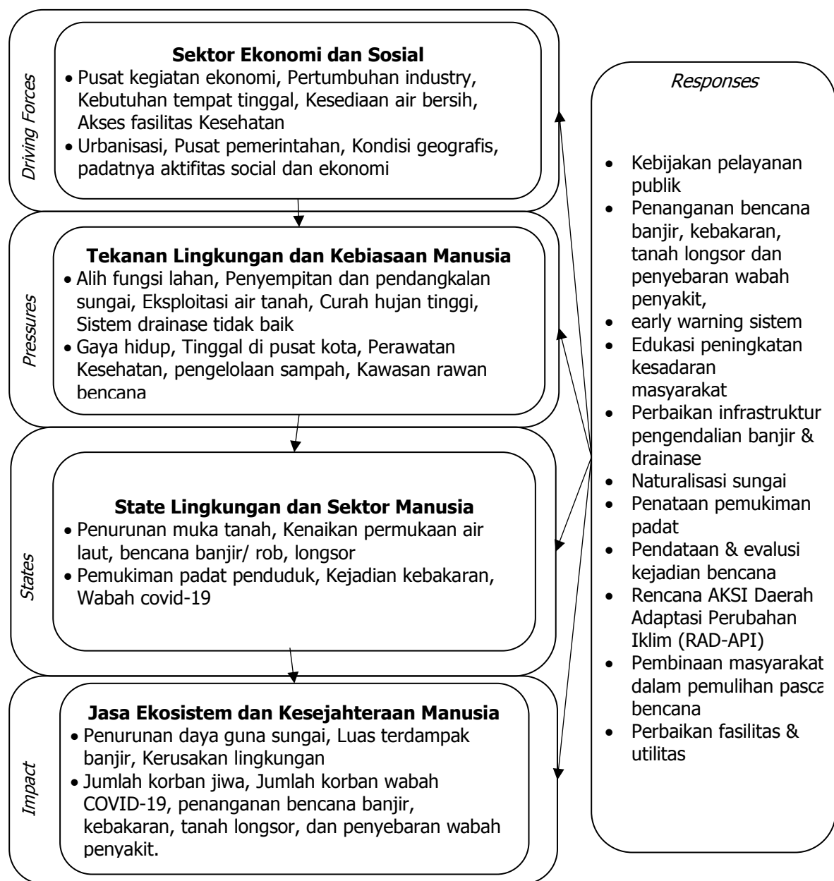
Gambar II-62 Konsep Analisis DPSIR Risiko Bencana
