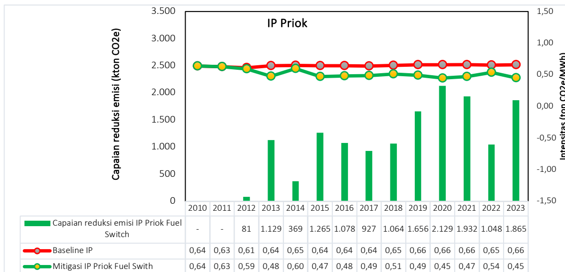
Gambar 4.22 Capaian penurunan emisi GRK dan intensitasnya di pembangkit Tanjung Priok
