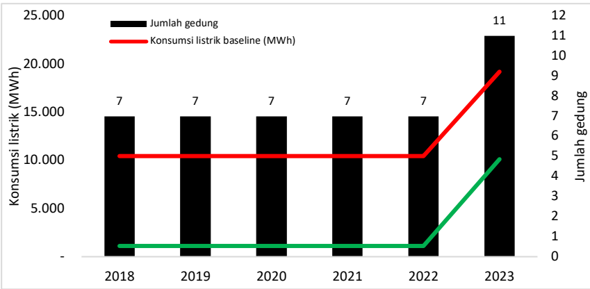
Gambar 4.13 Konservasi energi di gedung pemerintahan
