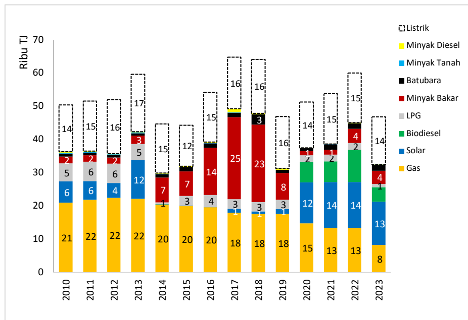
Gambar 3.16 Konsumsi energi sektor industri manufaktur
