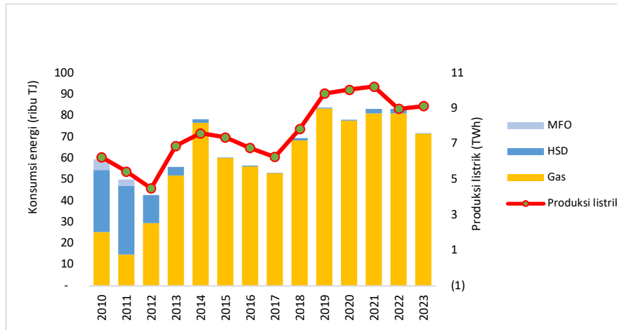
Gambar 4.5 Konsumsi bahan bakar di PT PLN Indonesia Power Tanjung Priok
