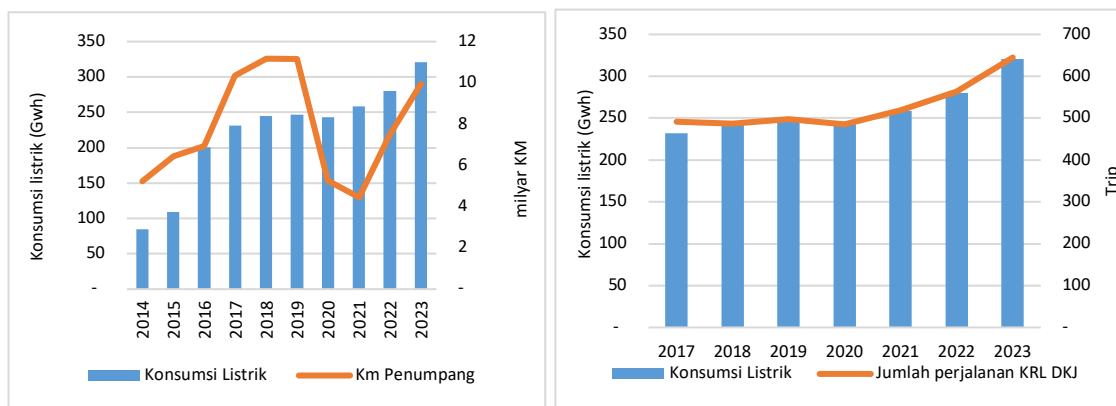
Gambar 4.9 (a) Konsumsi listrik, km-penumpang, dan (b) jumlah perjalanan dan konsumsi listrik KRL
