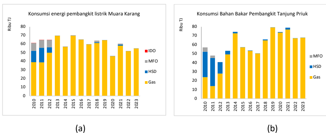
Gambar 3.15 Konsumsi energi di sektor pembangkit listrik: (a) PT PLN Nusantara Power Muara Karang dan (b) PT PLN Indonesia Power Priuk
