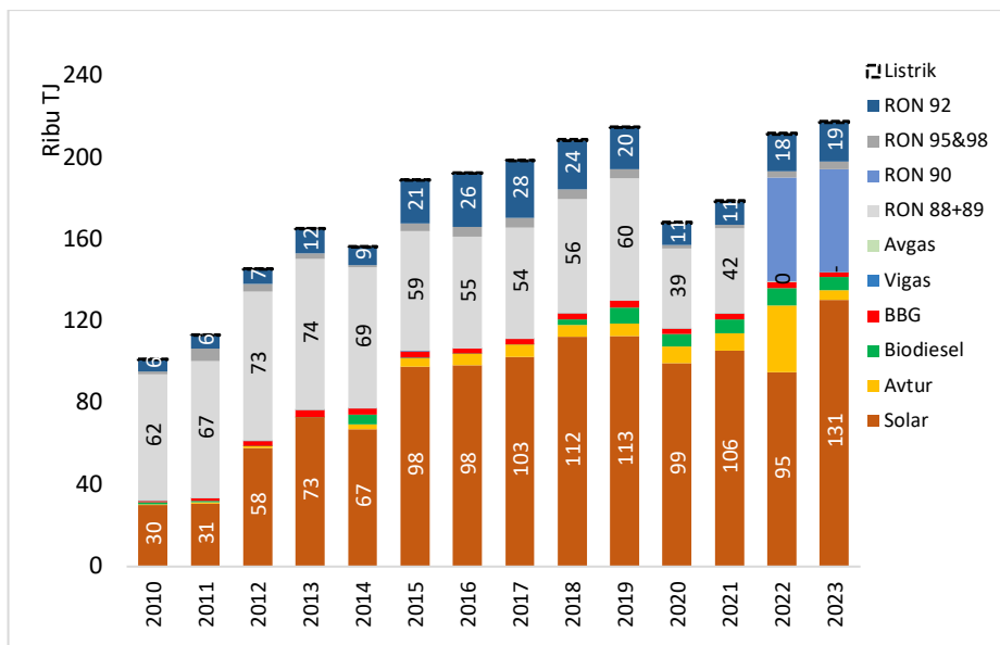
Gambar 3.17 Konsumsi energi sektor transportasi
