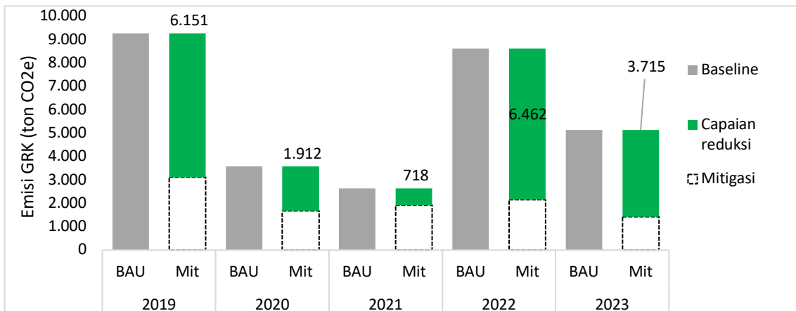
Gambar 4.28 Tingkat emisi GRK baseline, mitigasi dan capaian penurunan emisi GRK dari penggunaan kendaraan umum MRT
