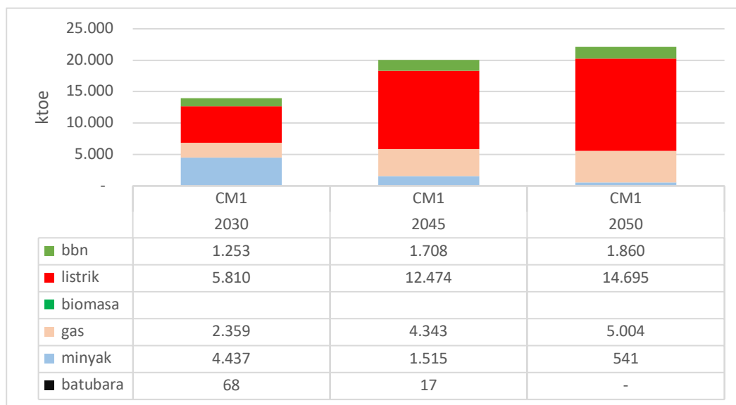
Gambar 5.16 Proyeksi kebutuhan energi 2030, 2045 dan 2050 berdasar jenis energi
