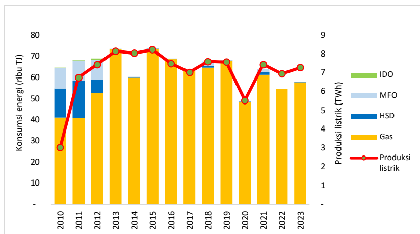
Gambar 4.4 Konsumsi bahan bakar di PT PLN Nusantara Power Muara Karang
