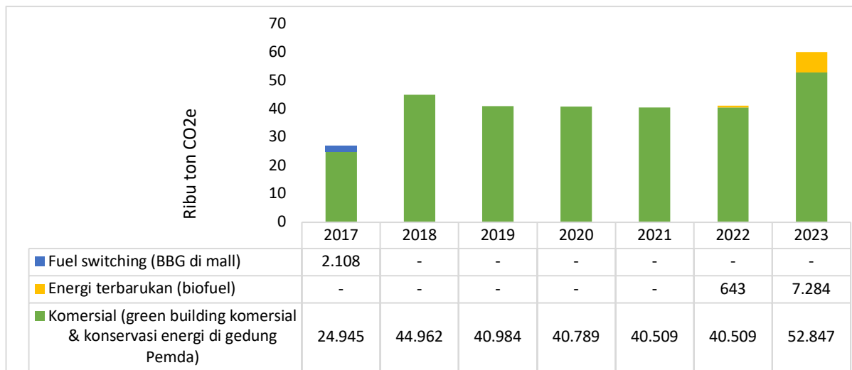
Gambar 4.30 Capaian penurunan emisi GRK di sub sektor bangunan
