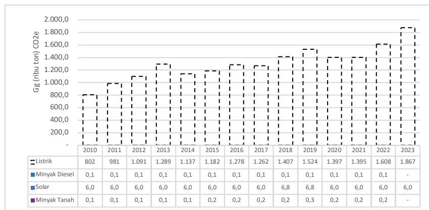
Gambar 3.35 Tingkat emisi GRK sektor lain-lain
