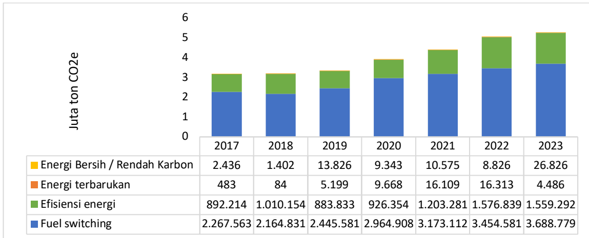
Gambar 4.20 Capaian penurunan emisi GRK di sub sektor pembangkit listrik
