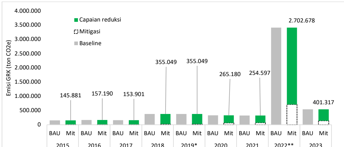
Gambar 4.25 Tingkat emisi GRK baseline, mitigasi dan capaian penurunan emisi GRK pada aksi mitigasi penggunaan kendaraan umum busway
