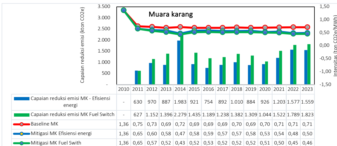
Gambar 4.21 Capaian penurunan emisi GRK dan intensitasnya di pembangkit Muara Karang
