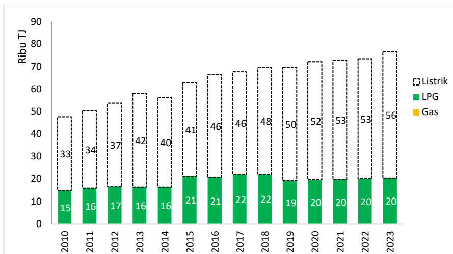
Gambar 3.19 Konsumsi bahan bakar dan pemakaian listrik sektor rumah tangga
